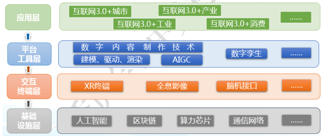
图 3 互联网 3.0 体系架构
